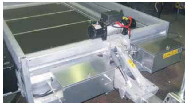
Elektrisk spil monteret på side panel, kan udstyres med fjernbetjening.
